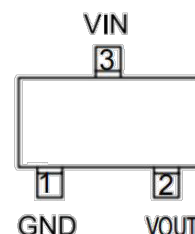
SOT23-3L & SOT23
